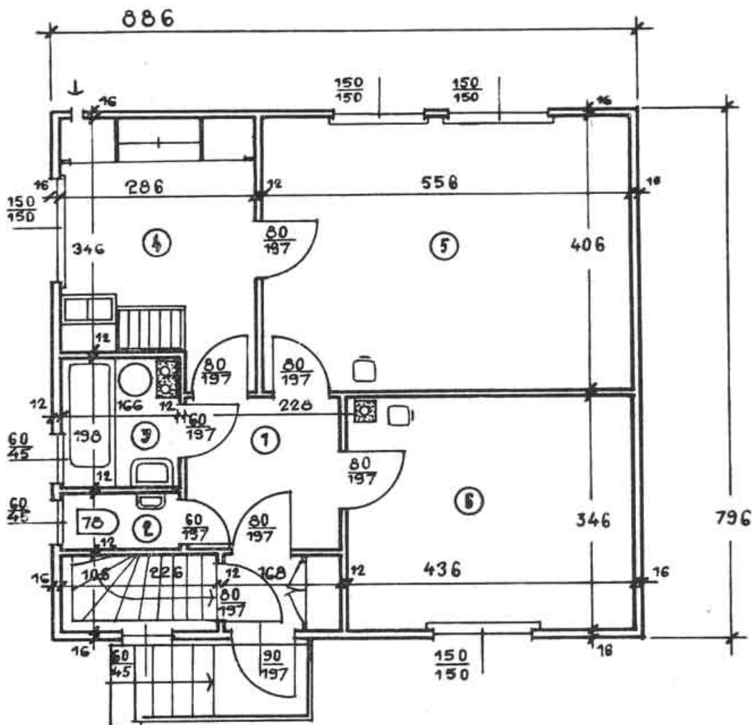
Obr. 6. Pôdorys dvojizbového bytu. 1 — predsieň, 2 — WC, 3 — kúpeľňa, 4 — kuchyňa, 5 — obývací izba, 6 — spálňa.
