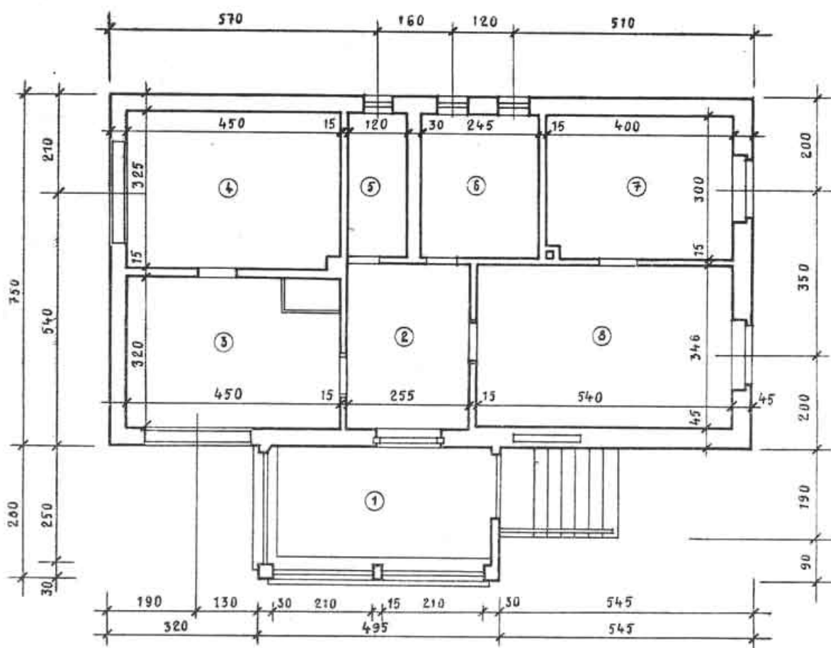
Obr. 4. Pôdorys prestavaného domu č. p. 367. 1 — veranda, 2 — predsieň, 3 — kuchyňa, 4 — spálňa rodičov, 5 — komora, 6 — kúpeľňa, 7 — spálňa detí, 8 — obývacia izba. Miestnosti č. 6, 7, a a polovica predsieni (2) tvoria pôvodný pôdorys jednoizbového domčeka (6 — komora, používaná väčšinou ako kuchyňa, 7 — izba — kuchyňa, používaná a zariadená ako izba).
